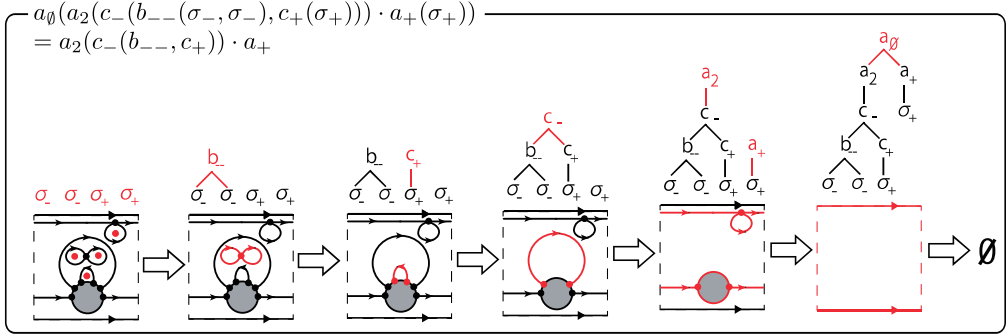
図 10. 流れの COT 表現の構成法の適用例
