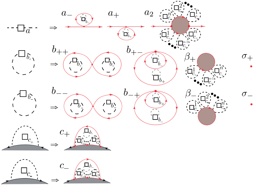
図 9. 流れのすべての構成要素
