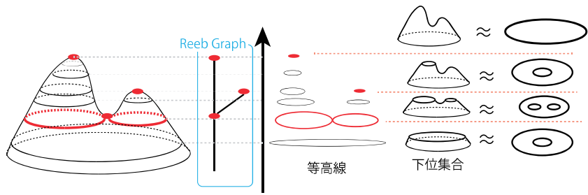
図 6. 山の等高線とその下位集合
