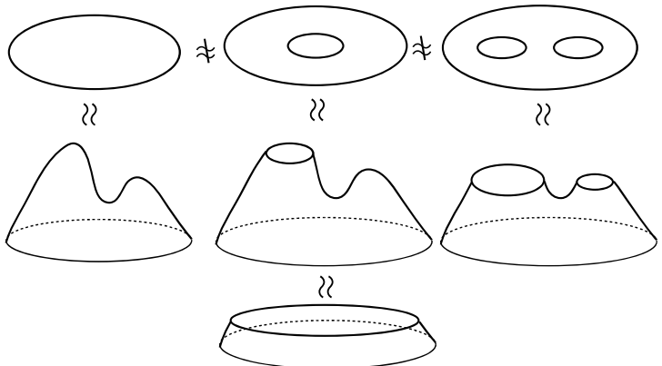
図 4. 円板 \not\sim 円環 \not\sim パンツ
