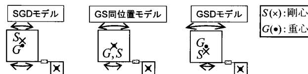
図 3 重心、剛心、連結ダンパーの位置関係による 3 つのモデル
