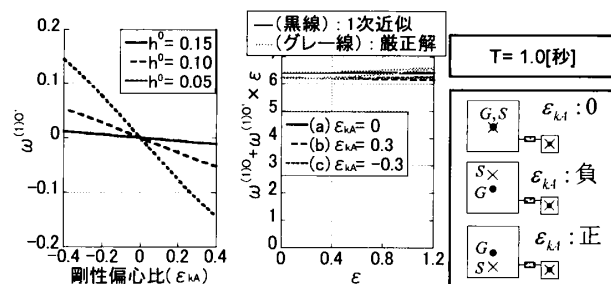
図 5 (左) 1 次固有円振動数の 1 階微係数 (右) 線形近似した 1 次固有円振動数と厳正解
