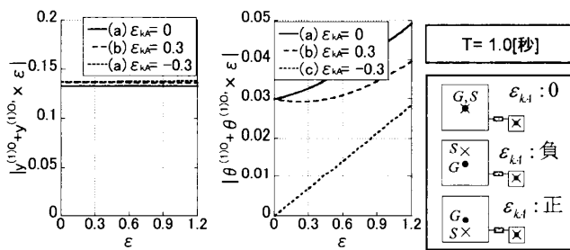
(a) 1 次並進成分 (b) 1 次ねじれ成分 図 6 1 次近似した 1 次モード成分の絶対値
